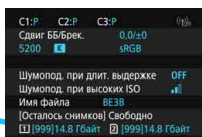
Настройки камеры
